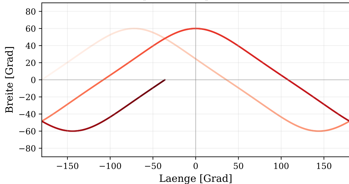
Abb. 6b: Bodenspur - Drosophila-Lemniskaten-Bahn
