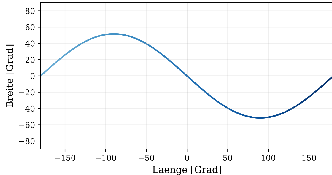
Abb. 6a: Bodenspur - Klassische LEO-Bahn (ISS-aehnlich)
