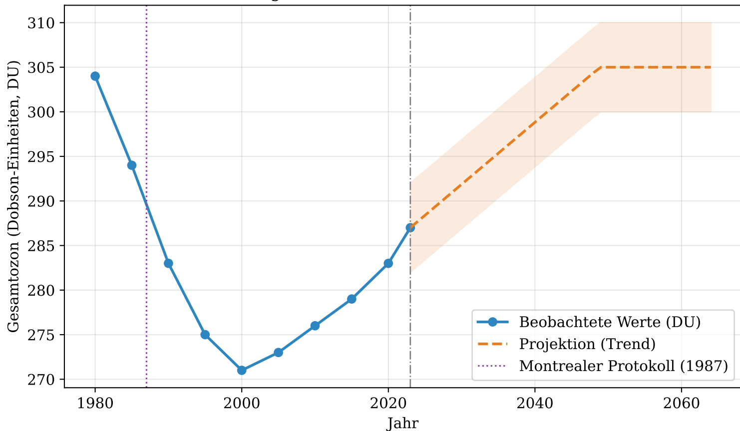
Plot 2 - Regeneration der Ozonschicht (1980-2060)
