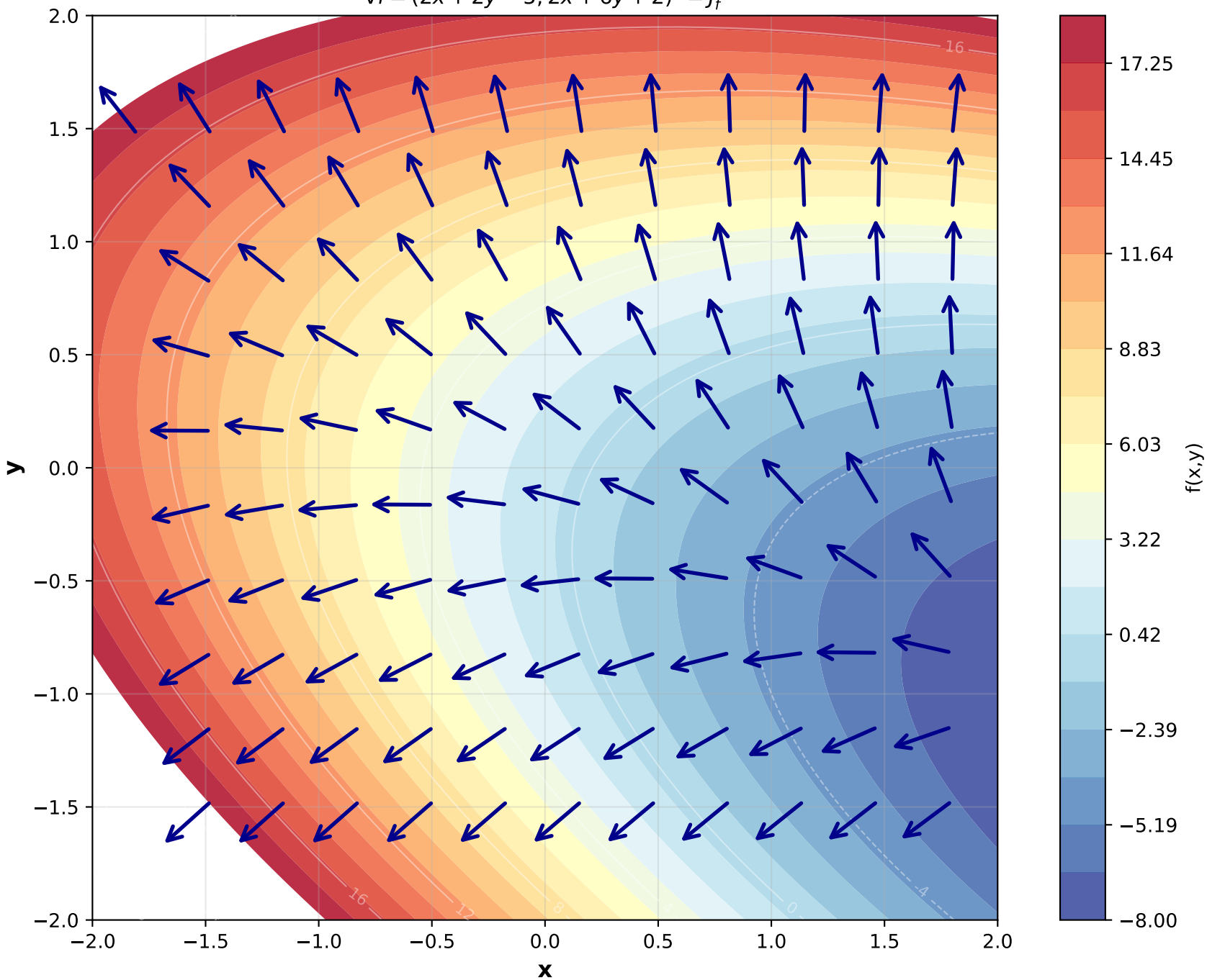
Plot 1: Quadratische Funktion mit Gradienten-Vektorfeld
