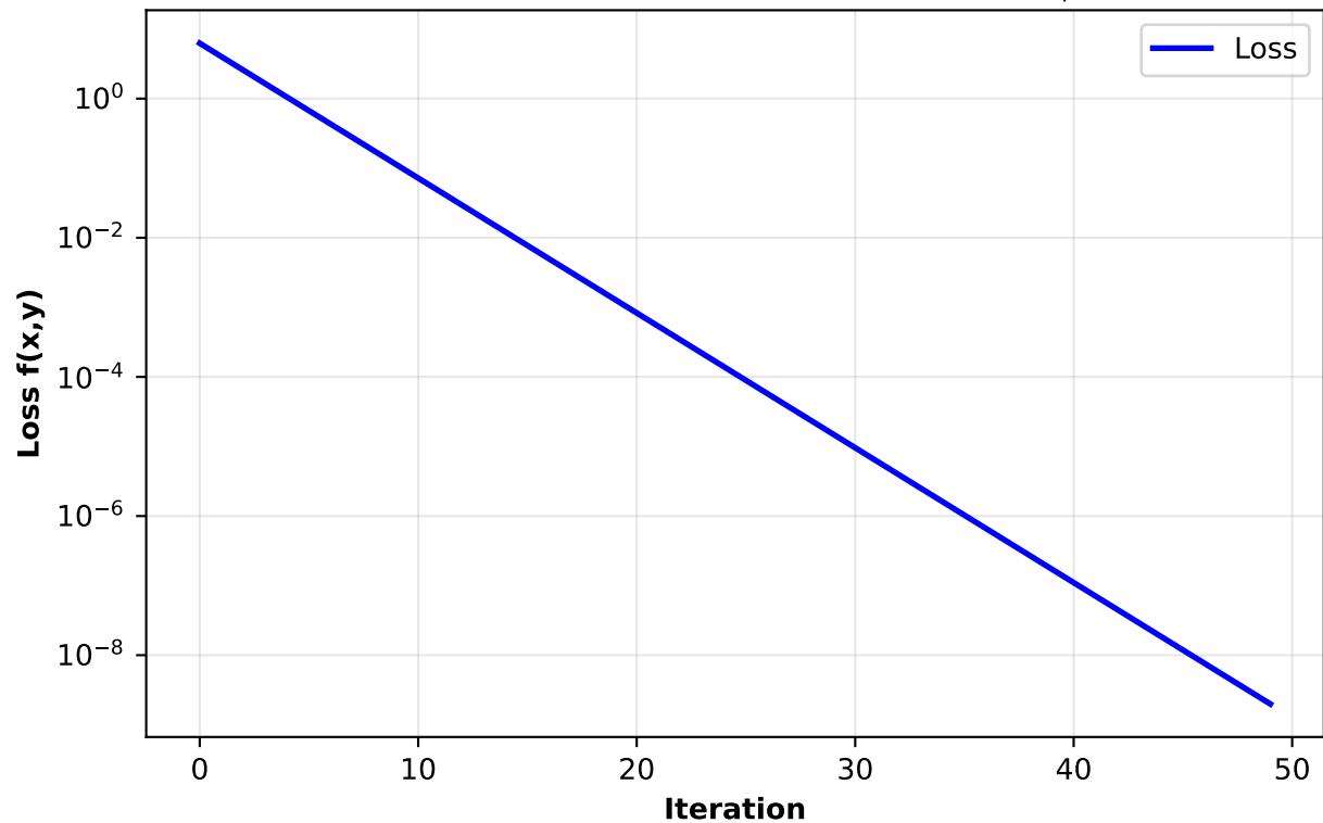
Konvergenz: x_{k+1} = x_k - \alpha \nabla f = x_k - \alpha J_f^T
