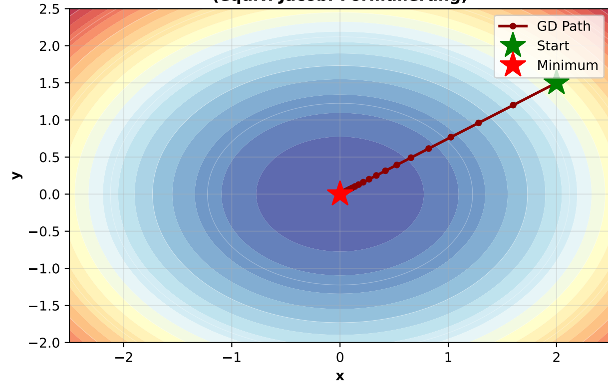
Gradientenabstieg-Pfad (equiv. Jacobi-Formulierung)
