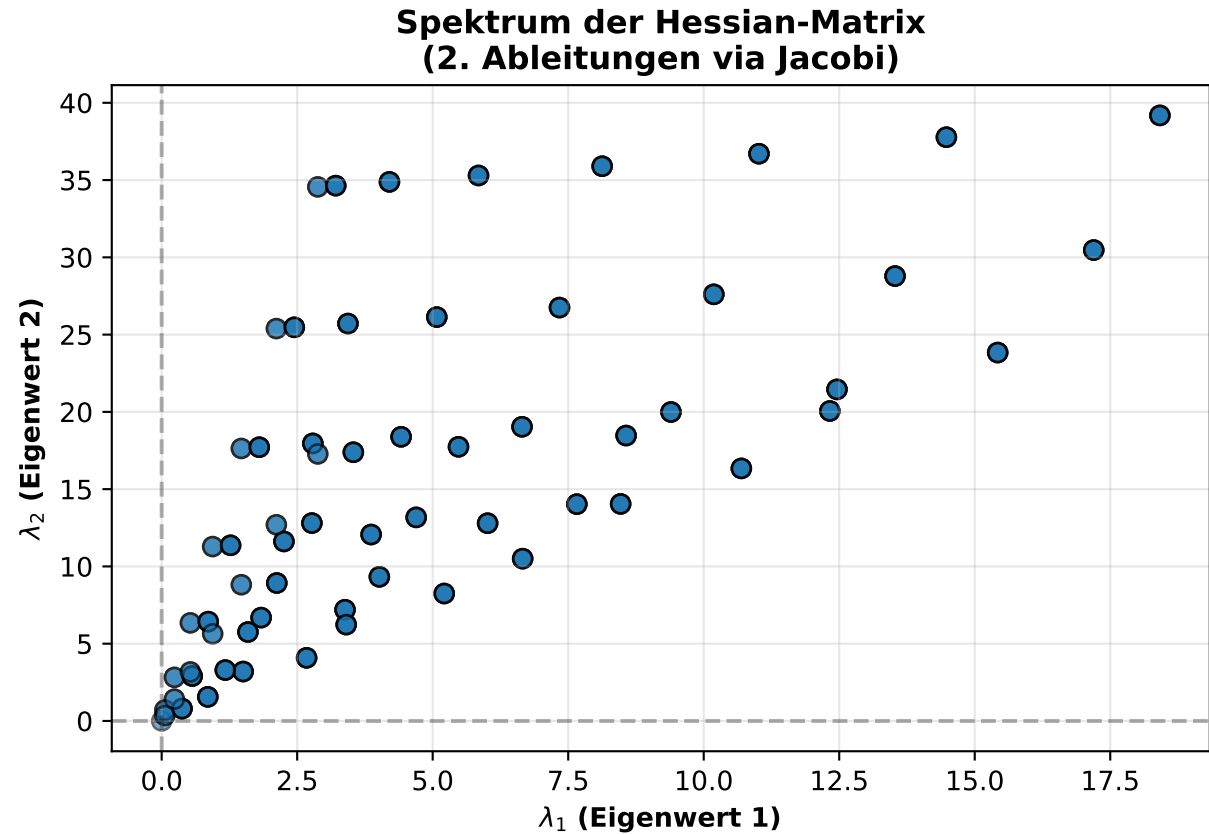
Plot 6: Spektralanalyse - Hessian als Jacobi-Struktur
