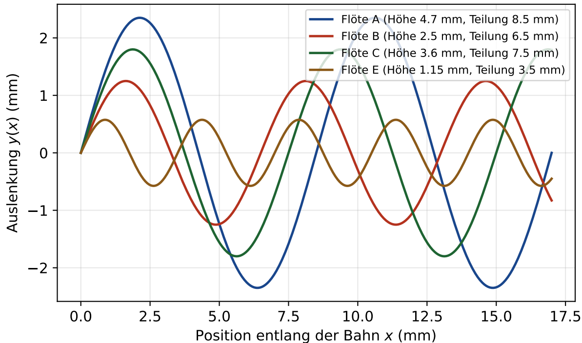
Sinusmodell der Flötenprofile gängiger Wellenarten
