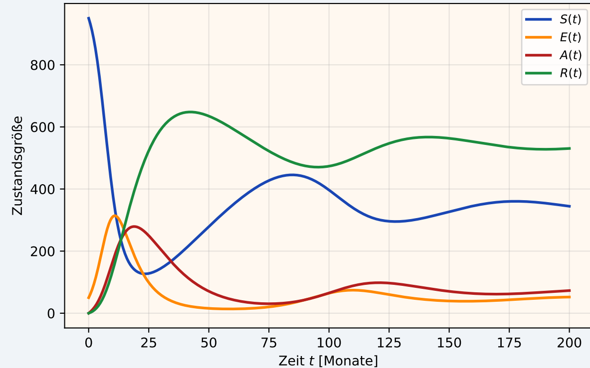
Szenario 3: Klimawandel
