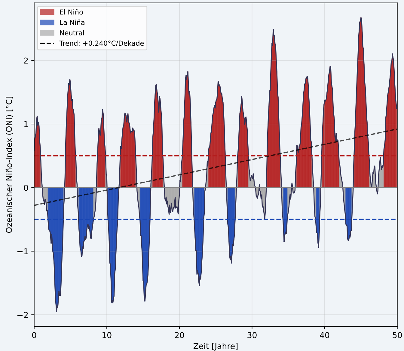
Simulierte ENSO-Zeitreihe (50 Jahre) El Niño / La Niña / Klimawandel-Trend
