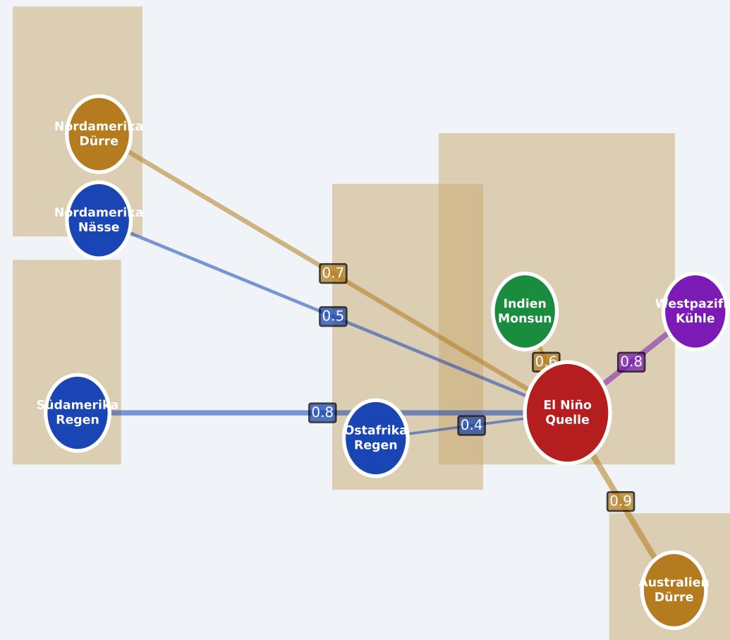
Globaler Telekonnectionsgraph G_{\text{ENSO}} (Kantengewichte = Korrelationsstärke)
