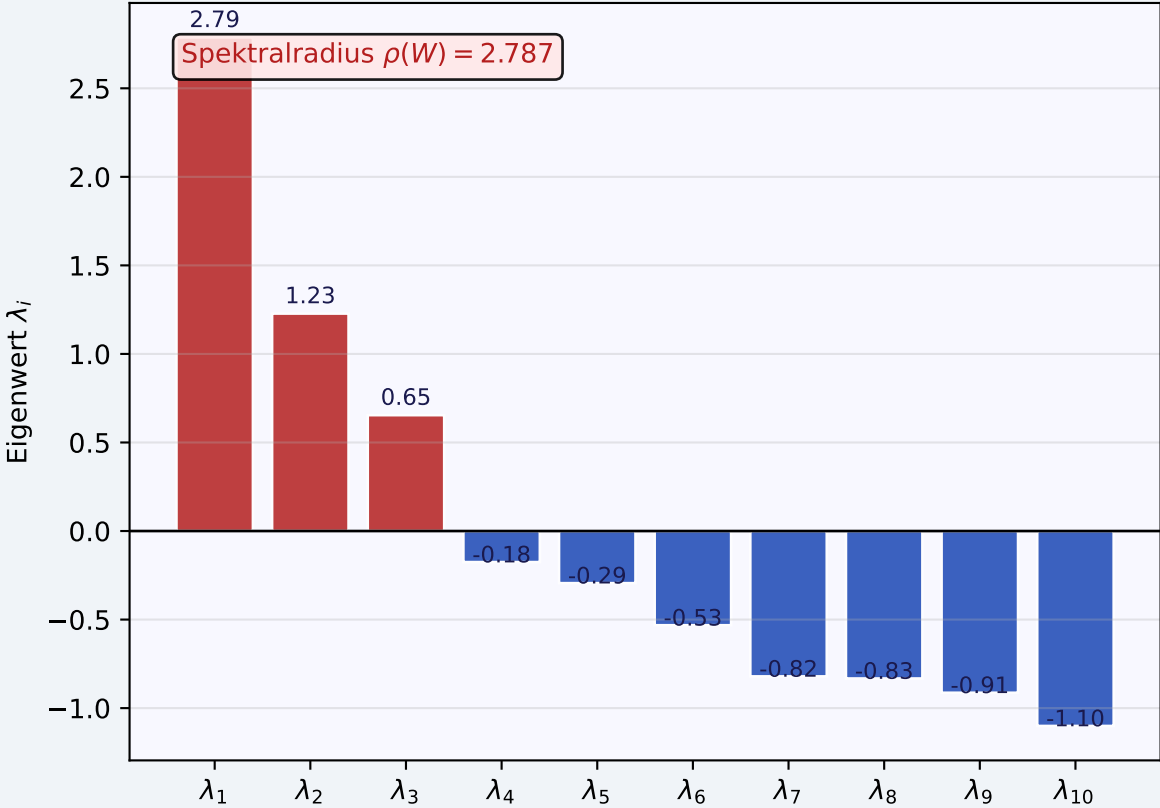
Eigenwertspektrum von W (spektrale Stabilitätsanalyse)
