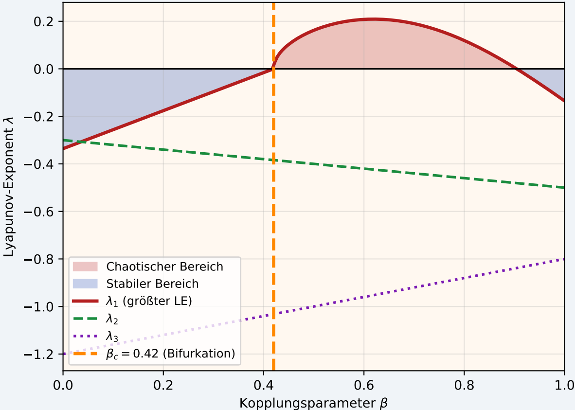
Lyapunov-Spektrum des Klimasystems (Stabilitätsbifurkation bei \beta_c )
