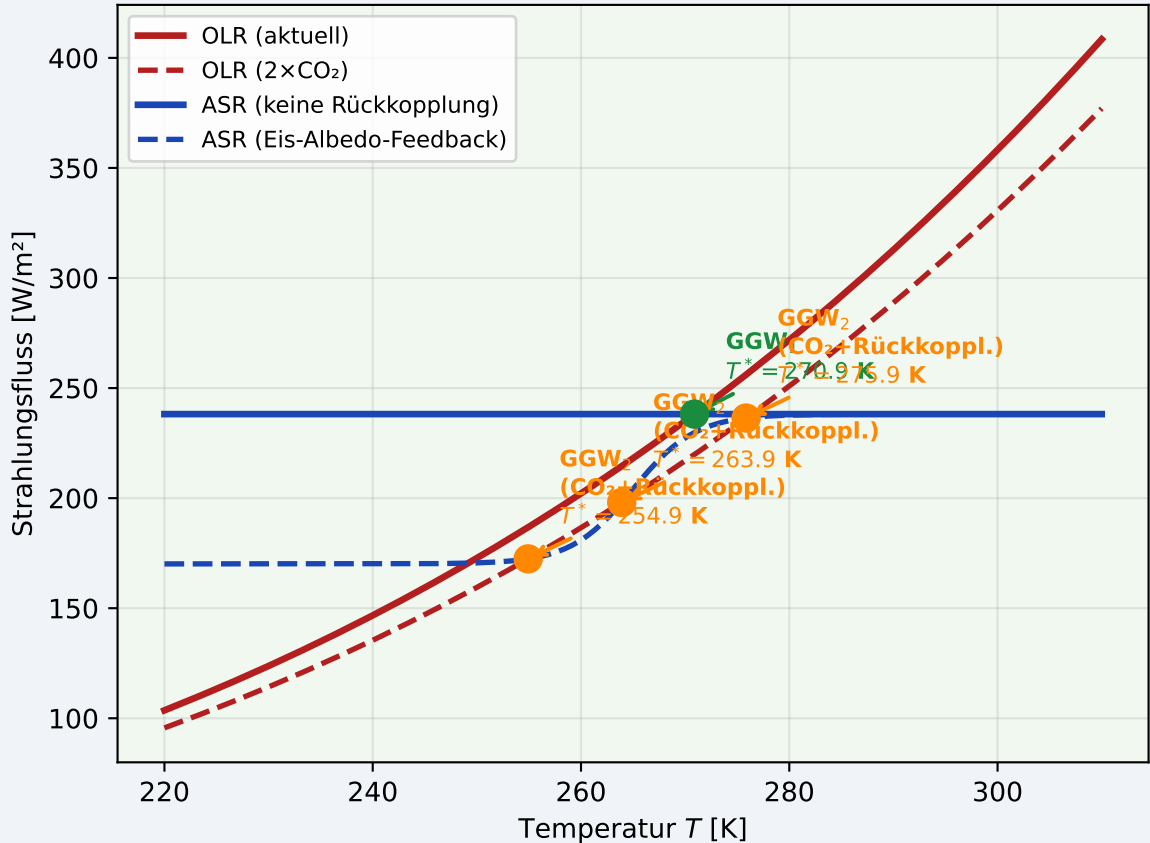
Strahlungsbilanz und Gleichgewichtstemperaturen (Rückkopplungsmechanismen)
