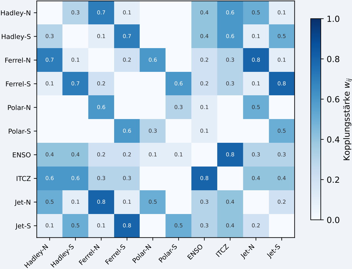
Gewichtete Adjazenzmatrix W des Klimagraphen G_{\text{klima}}
