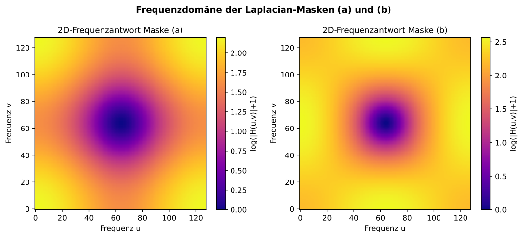
Figure 8: 2D-Frequenzantwort der Masken (a) und (b) (logarithmisch skaliert, hellere Bereiche = stärkere Antwort). Beide Masken zeigen klares Hochpassverhalten: Die Energie konzentriert sich bei hohen Frequenzen (Randbereiche). Maske (b) zeigt eine rundere Hochpasscharakteristik – konsistent mit ihrer besseren Rotationsinvarianz. Bildverarbeitungsbedeutung: Kanten entsprechen hohen Ortsfrequenzen. Die Masken verstärken genau diese Frequenzen und dämpfen Gleichanteile.
