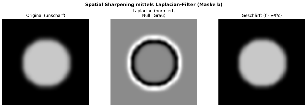
Figure 7: Spatial Sharpening in der Bildverarbeitung. Links: Unscharfes Originalbild. Mitte: Laplacian-Ausgabe (normiert, Null = Mittelgrau) – zeigt ausschließlich Kantenbereiche. Rechts: Geschärftes Bild I_s = I - \nabla^2 I/c . Kanten und Objektgrenzen sind deutlich verstärkt, homogene Bereiche bleiben unverändert. Praktischer Nutzen: Diese Methode wird eingesetzt in Druckvorverarbeitung, Kamerasoftware (Schärfereglern), medizinischer Bildgebung und Satellitenbildbearbeitung.
