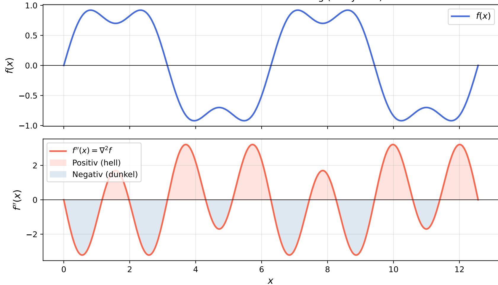
Funktion und ihre zweite Ableitung (analytisch)
