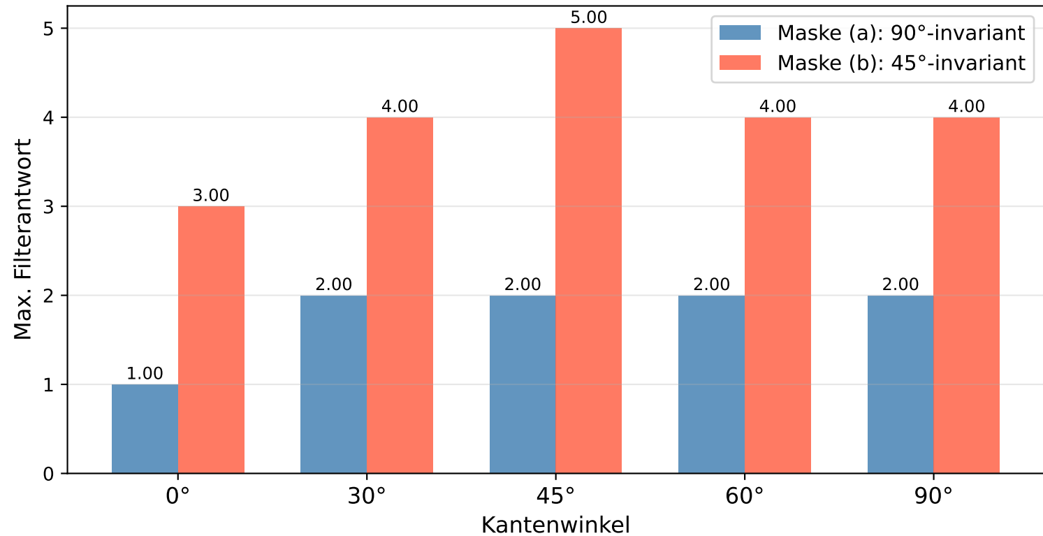
Rotationsinvarianz: Maximale Filterantwort bei verschiedenen Kantenorientierungen
