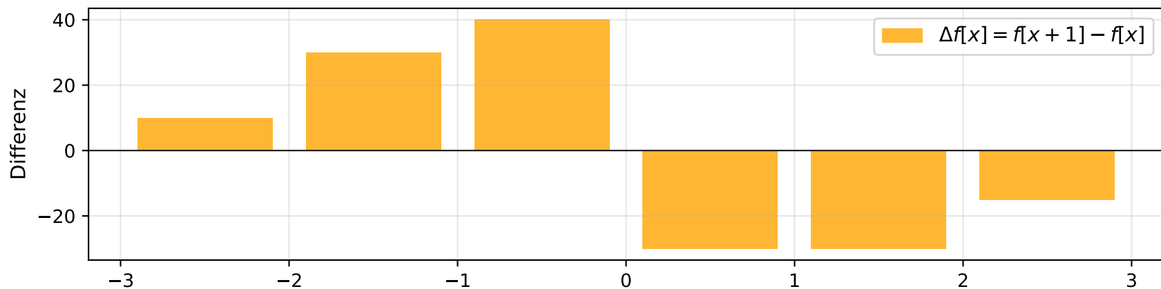
Erste diskrete Differenz \Delta f[x]
