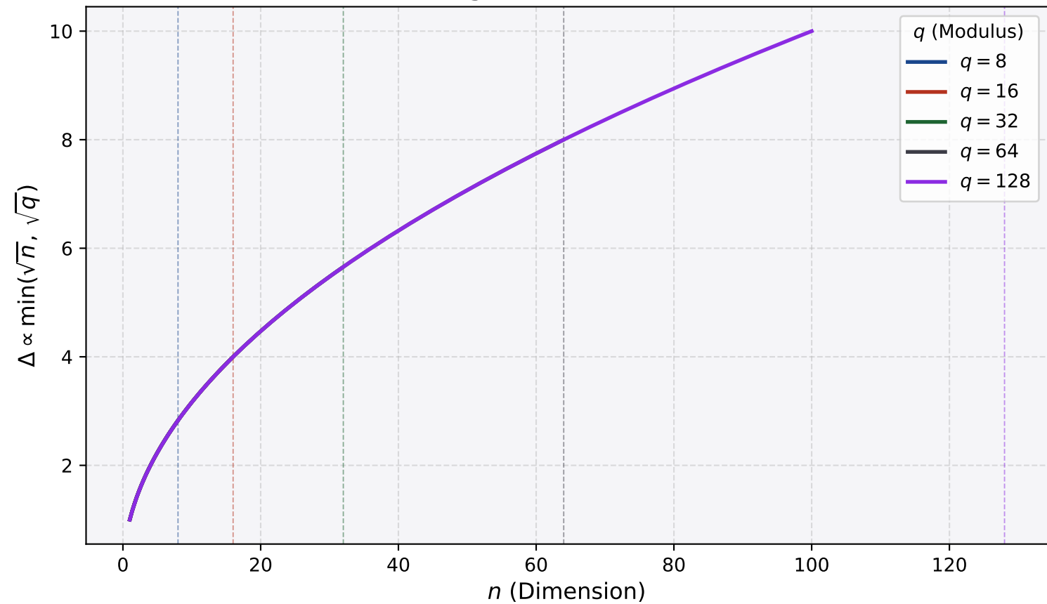
GKP Code-Distanz (Ring-SIS Konstruktion) nach Poster-Formel
