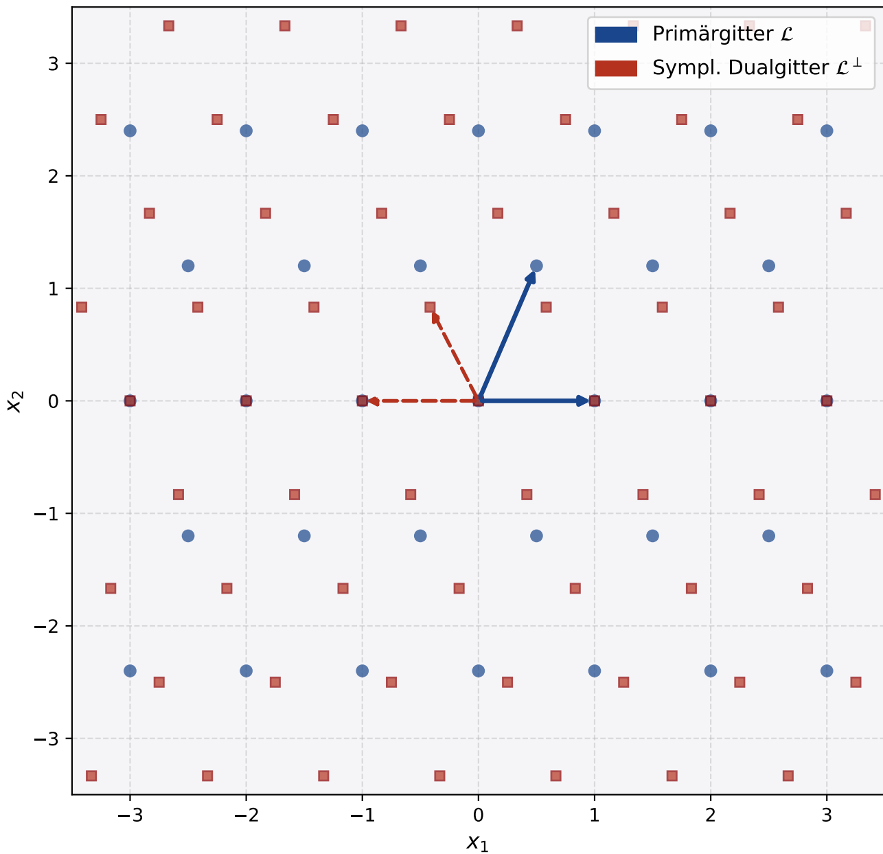
Primärgitter \mathcal{L} und symplektisches Dualgitter \mathcal{L}^\perp
