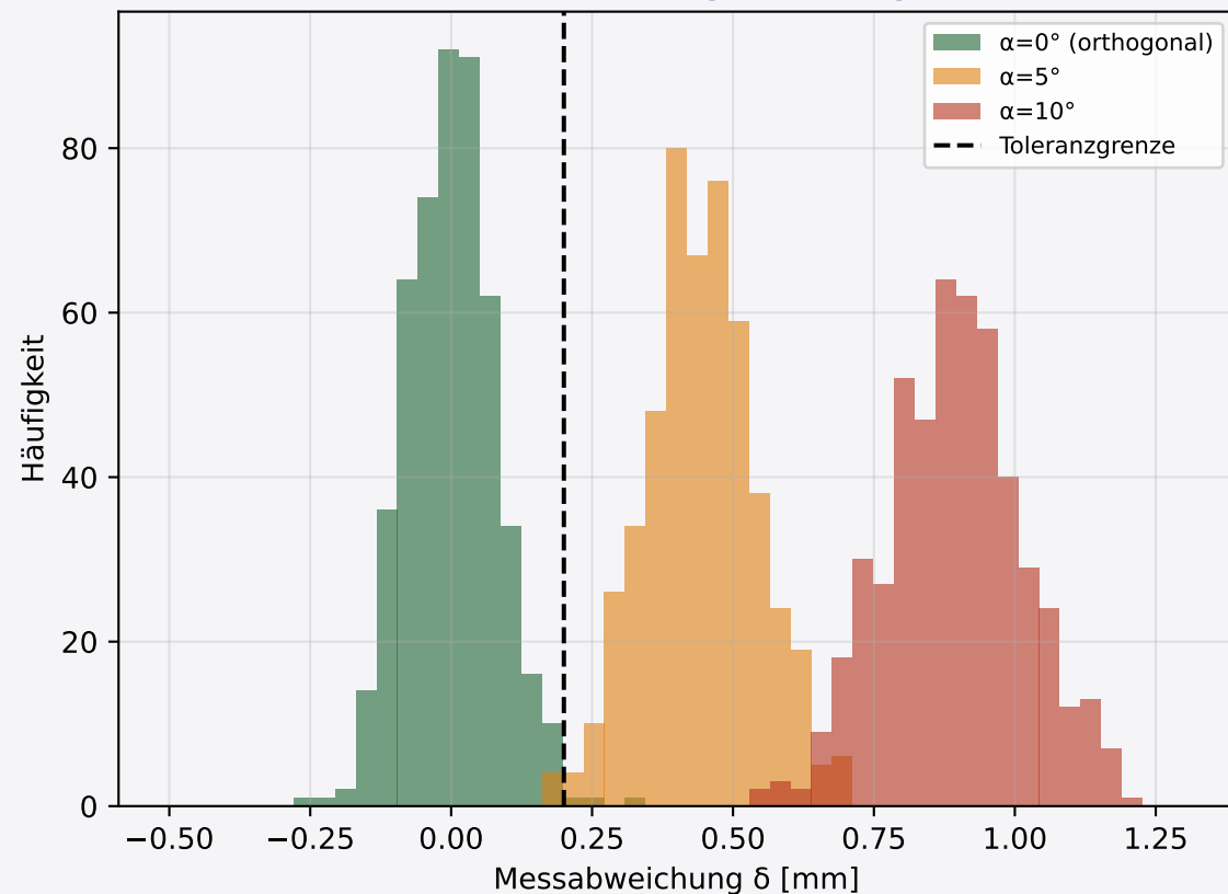
Messabweichungsverteilung
