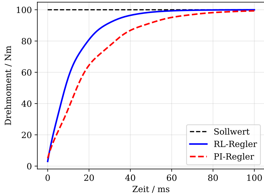
Sprungantwort RL vs. PI
