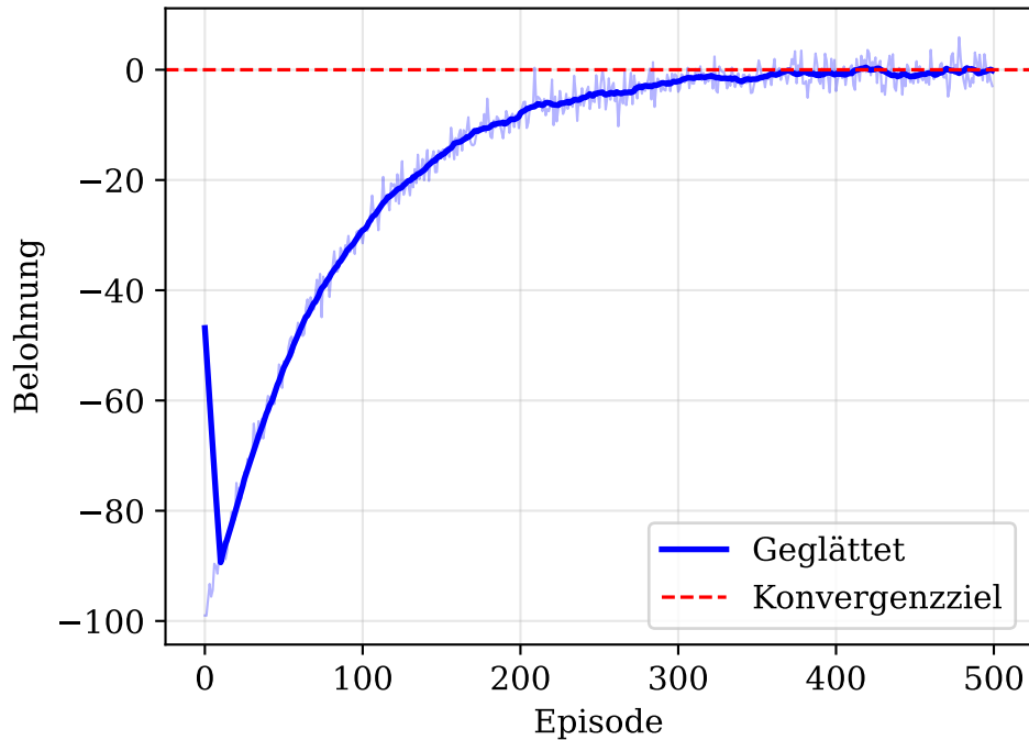
RL Trainingskonvergenz
