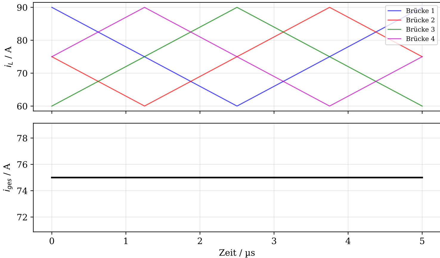
4 phasenversetzte Halbbrücken (GaN, 200 kHz)
