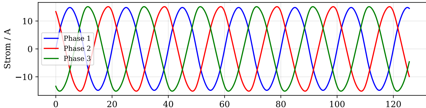
Dreiphasig ohne PFC
