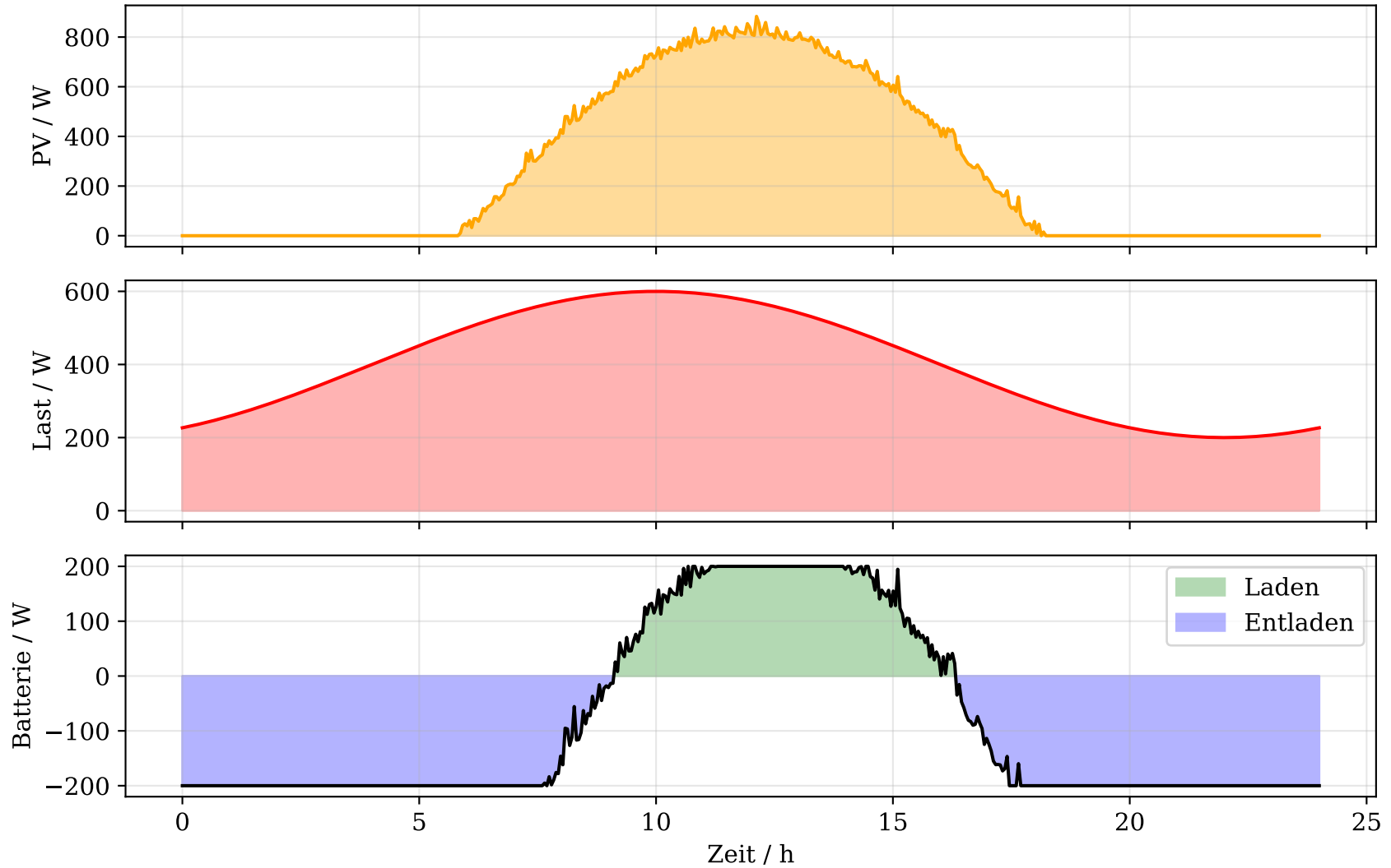
Microgrid 24h: PV, Last, Batterie
