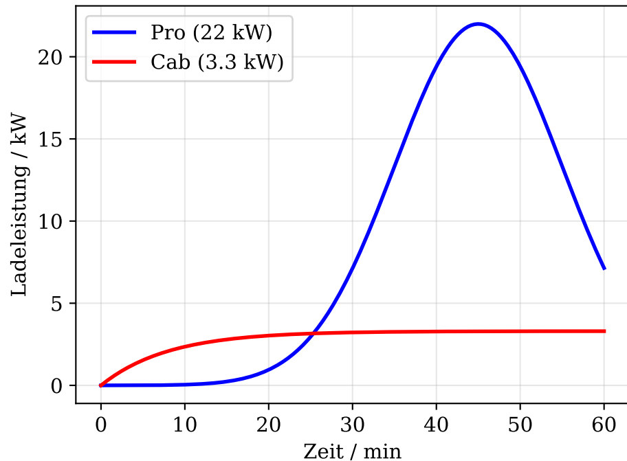
NeMo.bil Ladeverlauf Konvoi
