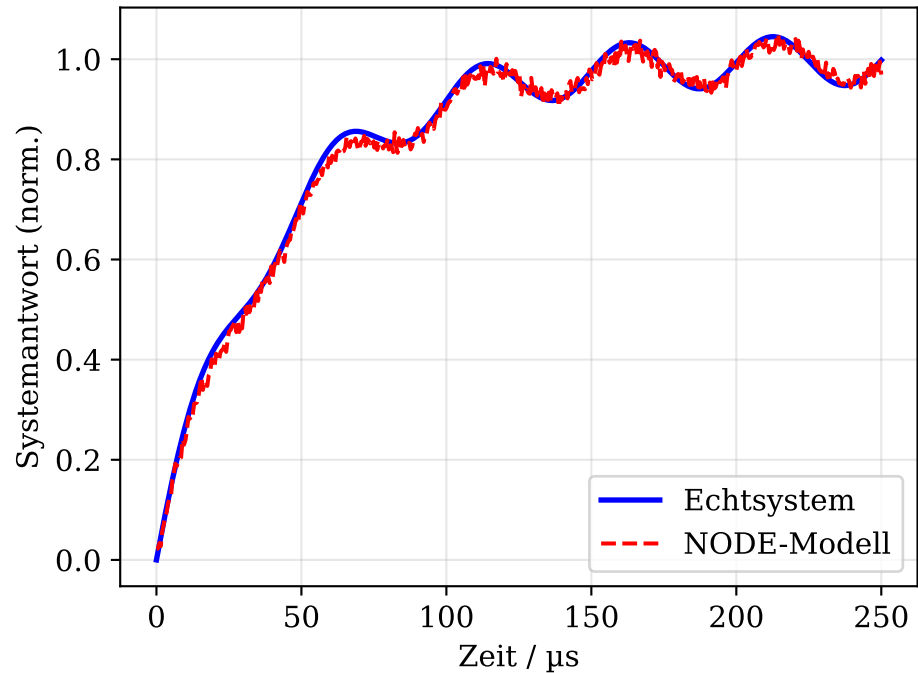
ML-Expert: NODE vs. Echtsystem
