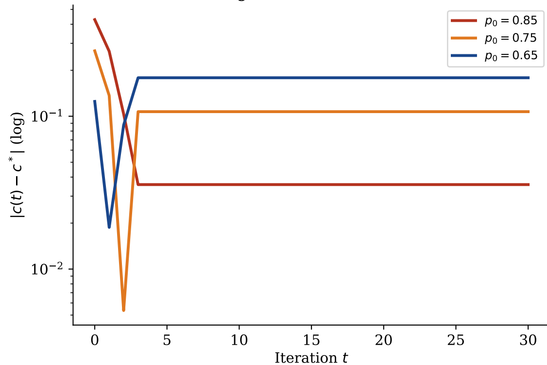
(b) Konvergenzgeschwindigkeit (logarithmische Skala)
