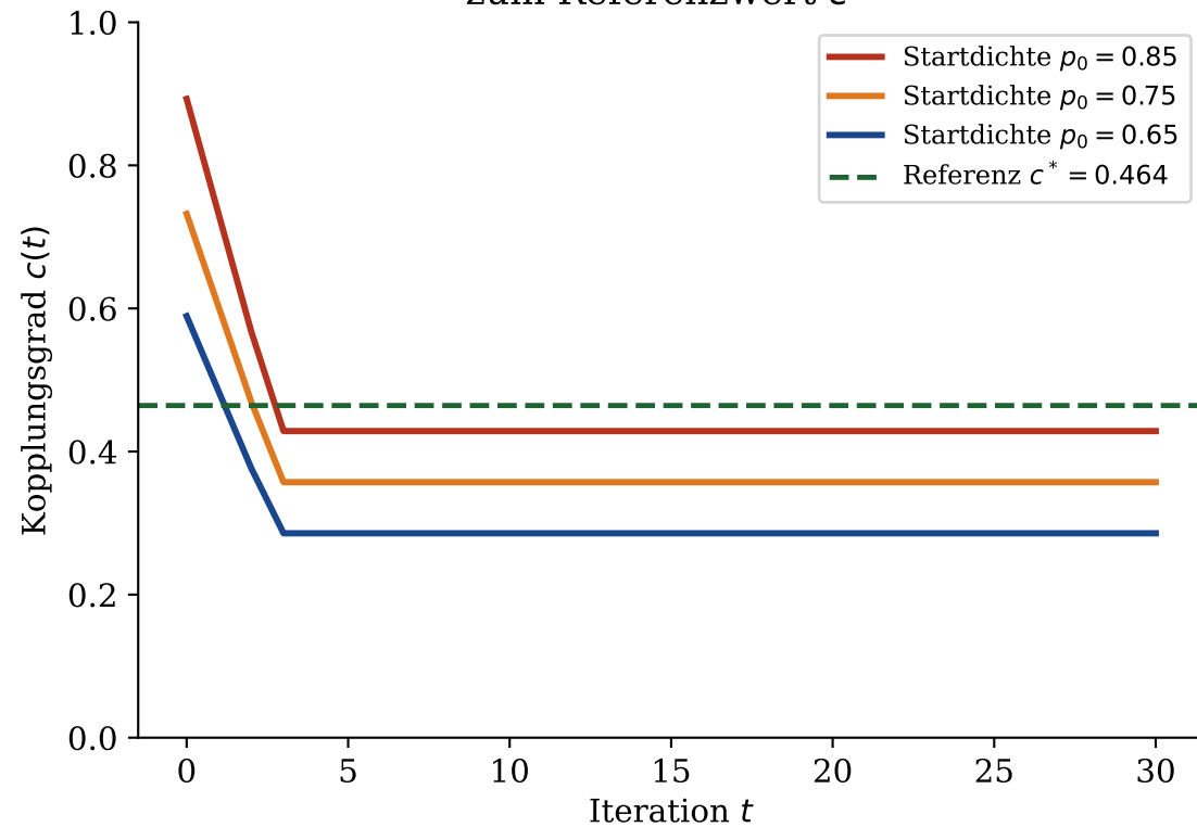
(a) Konvergenz des Kopplungsgrades zum Referenzwert c^*
