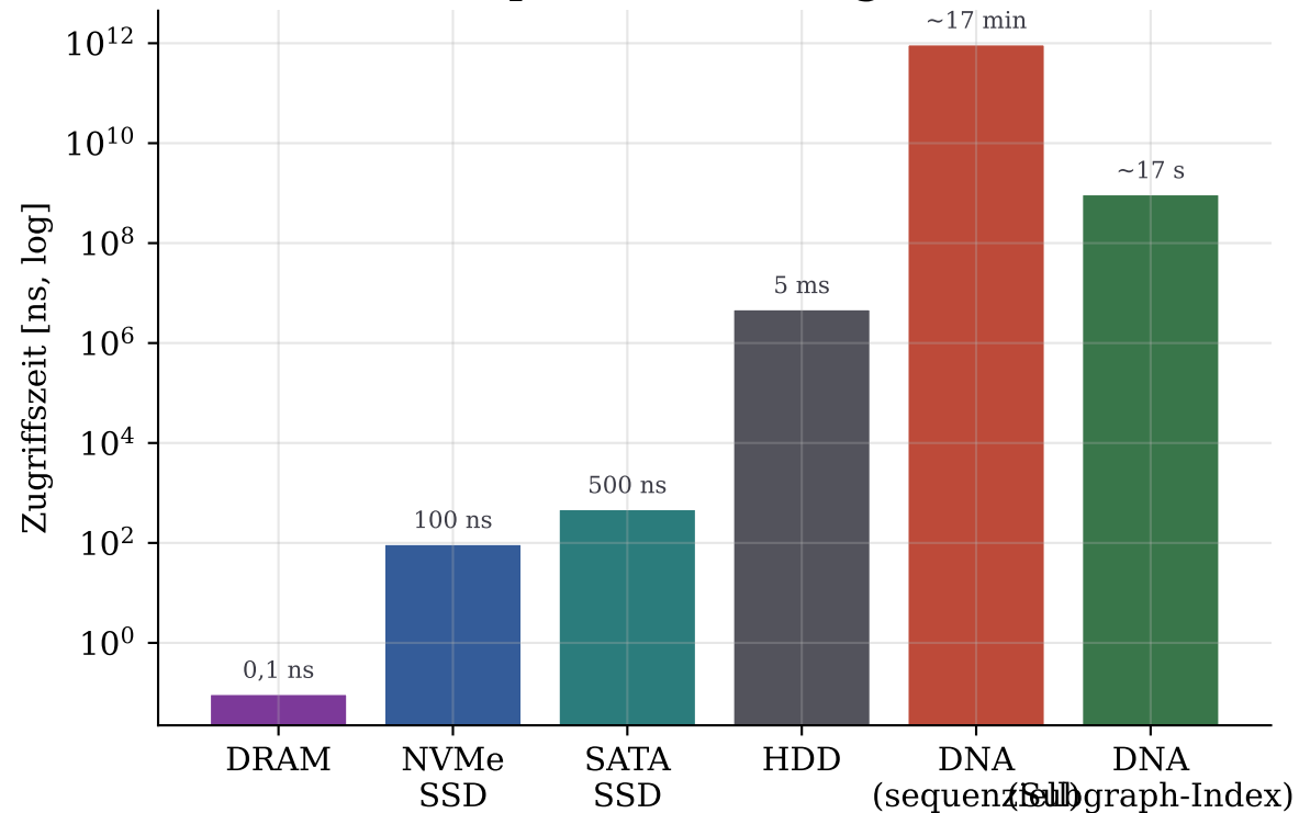
Zugriffszeit verschiedener Speichertechnologien
