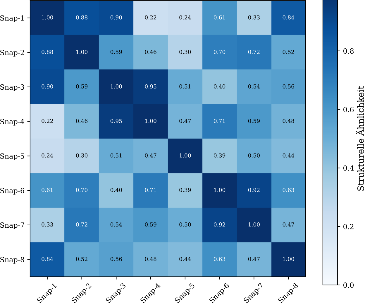
Subgraph-Ähnlichkeitsmatrix: Btrfs-Snapshots
