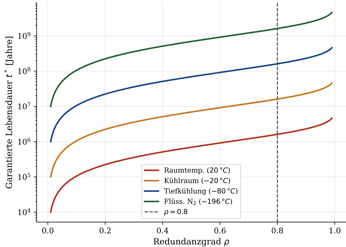
Garantierte Lebensdauer t^* = -\ln(1 - \rho)/\lambda
