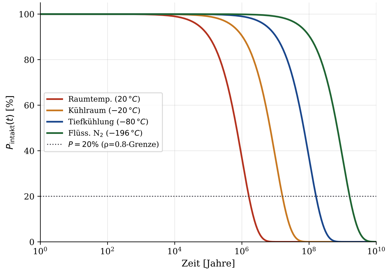
Haltbarkeitsmodell: P_{\text{intakt}}(t) = e^{-\lambda t}
