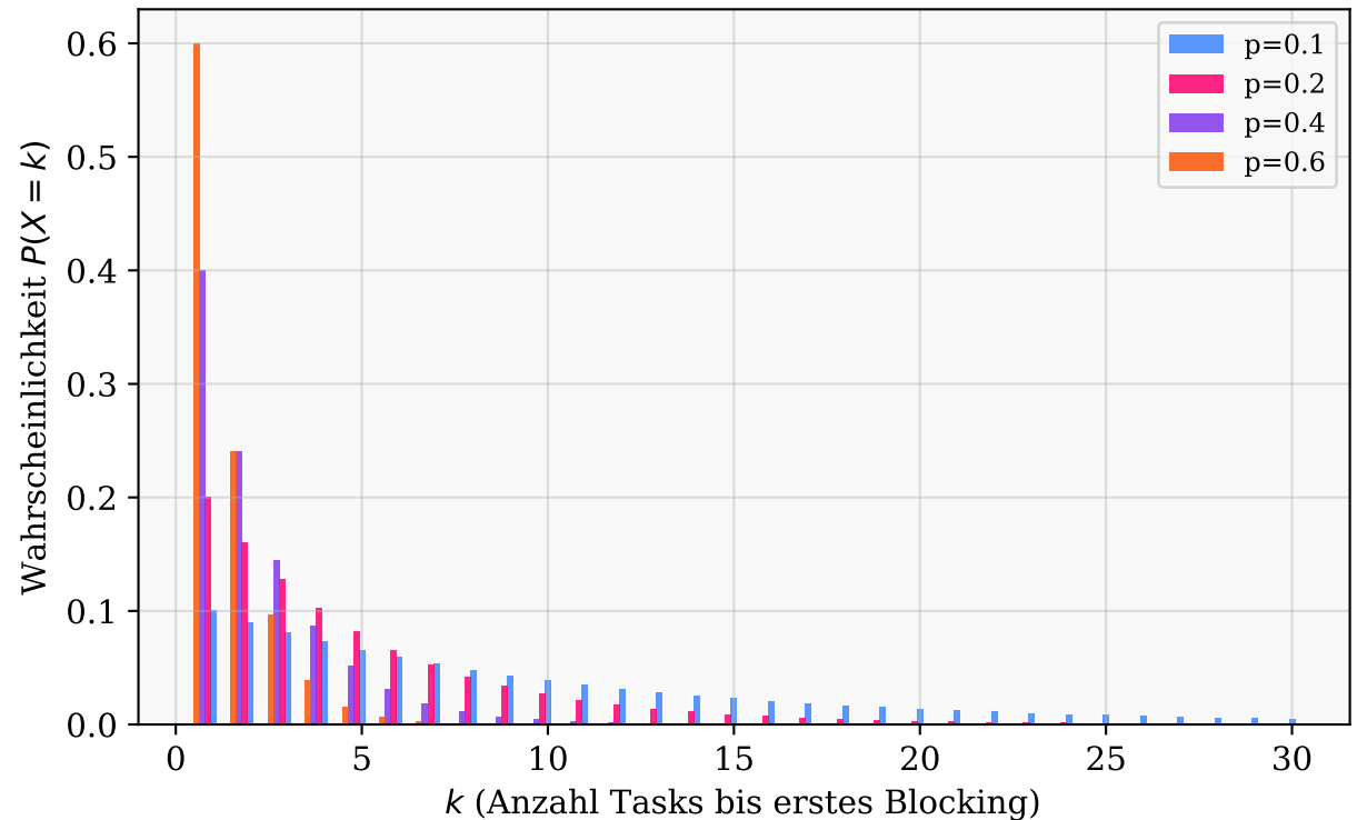
PMF der Geometrischen Verteilung
