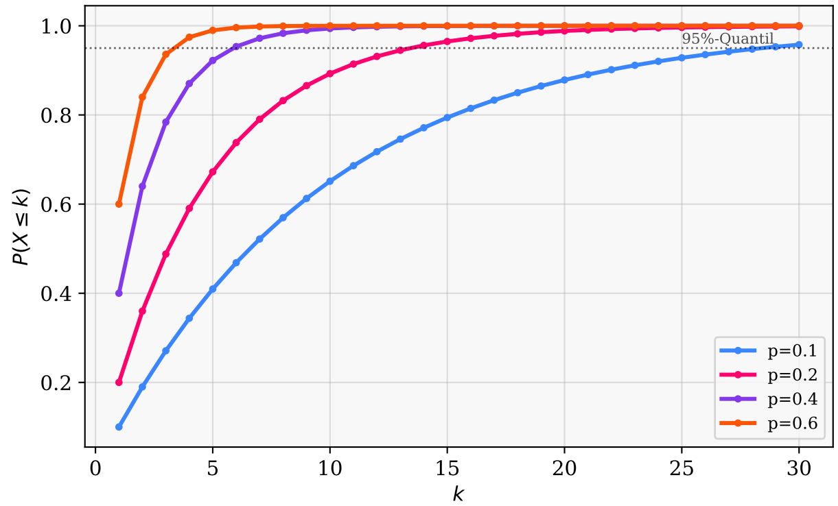
CDF der Geometrischen Verteilung
