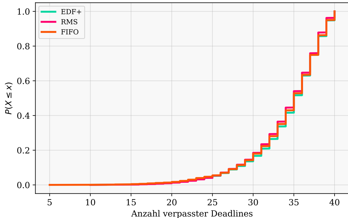
Empirische CDF: Stochastische Dominanz von EDF+
