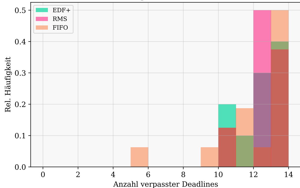
Histogramm: Verpasste Deadlines (N=40, p=0.15, 5000 Sim.)
