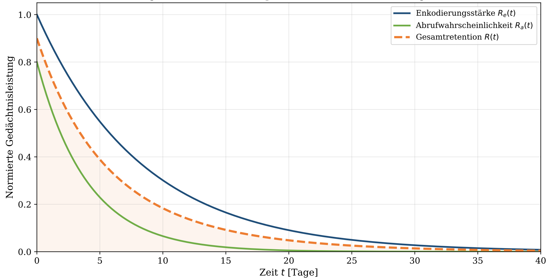
Abbildung 3: Bidirektionales Exponentialmodell – Enkodierung vs. Abruf
