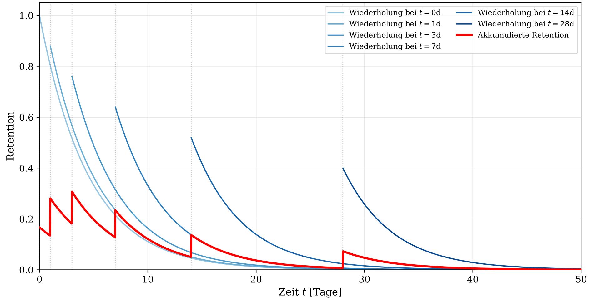
Abbildung 4: Spaced Repetition - Superposition exponentieller Zerfälle
