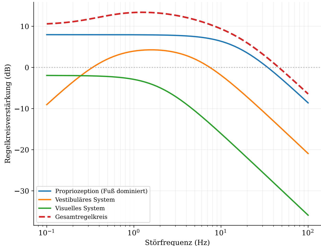
Bode-Diagramm: Posturaler Regelkreis (Frequenzgang der Sensormodule)
