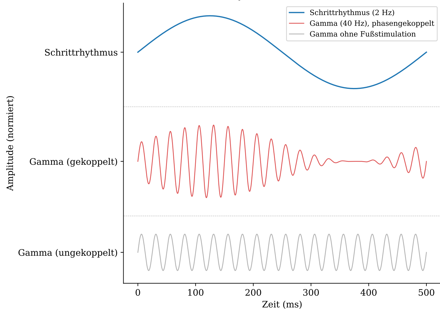
Phase-Amplitude-Kopplung: Schrittrhythmus → Gamma-Aktivität
