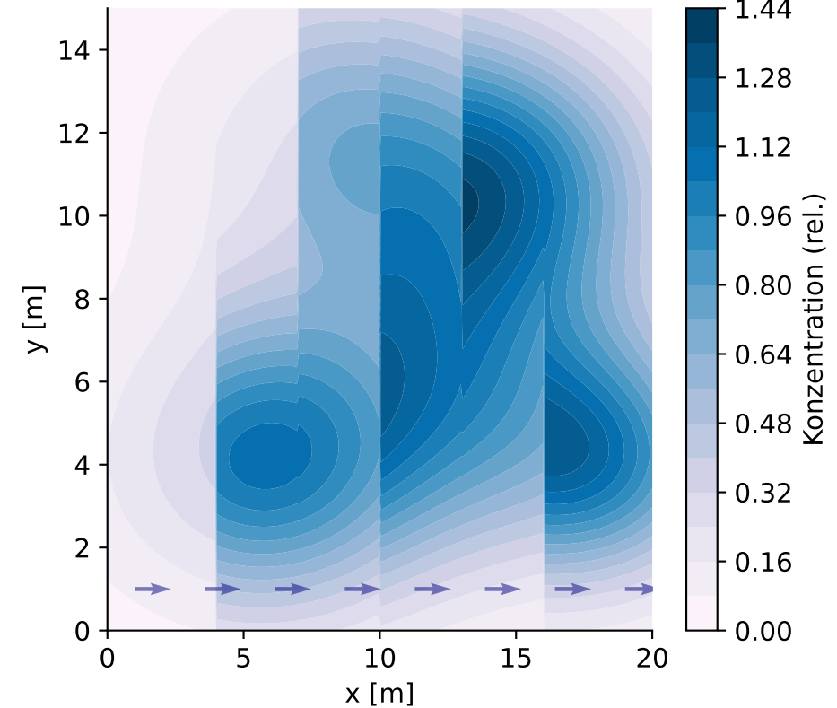
Windverwehte Duftwolken
