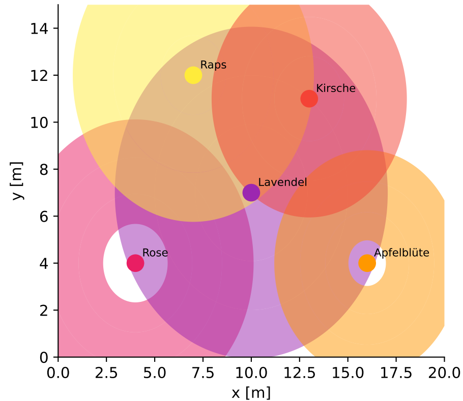
Einzelne Duftstofffelder
