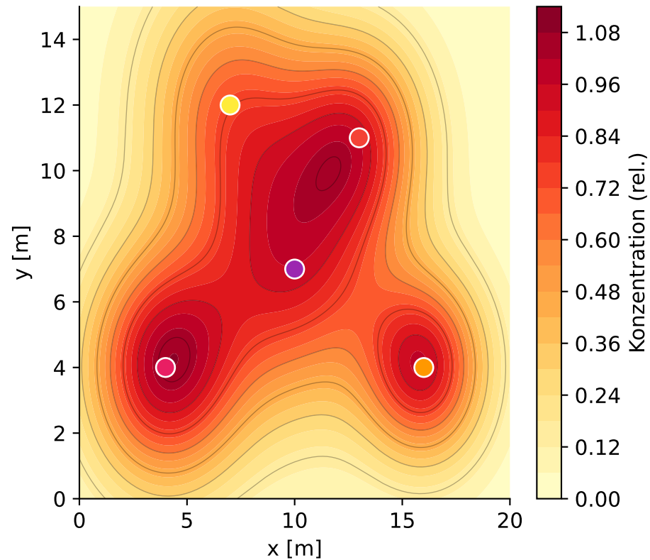
Summiertes Duftstofffeld
