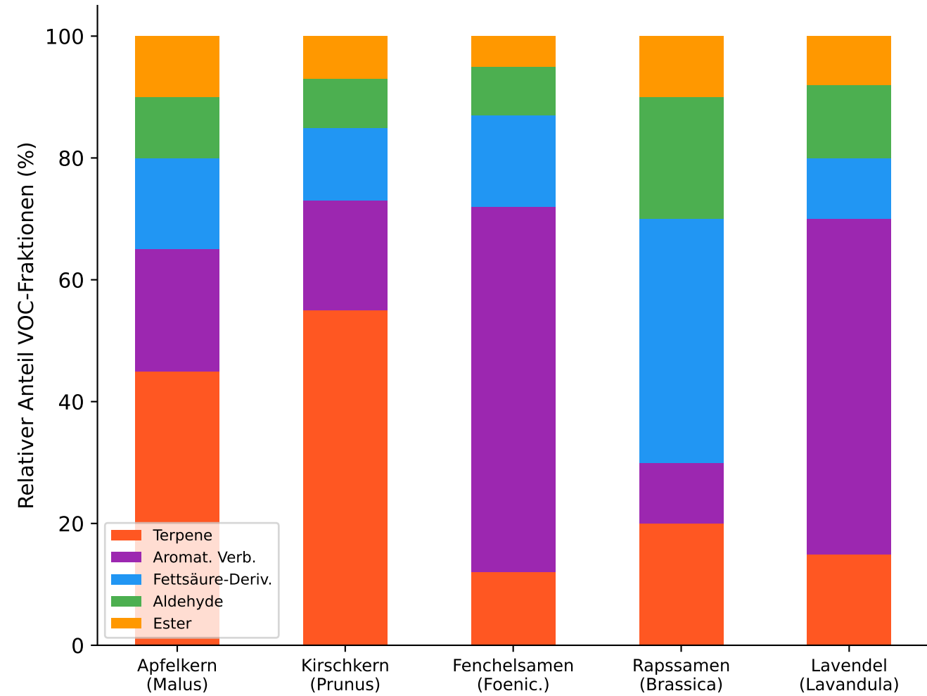
VOC-Klassen in ausgewählten Samenkernen
