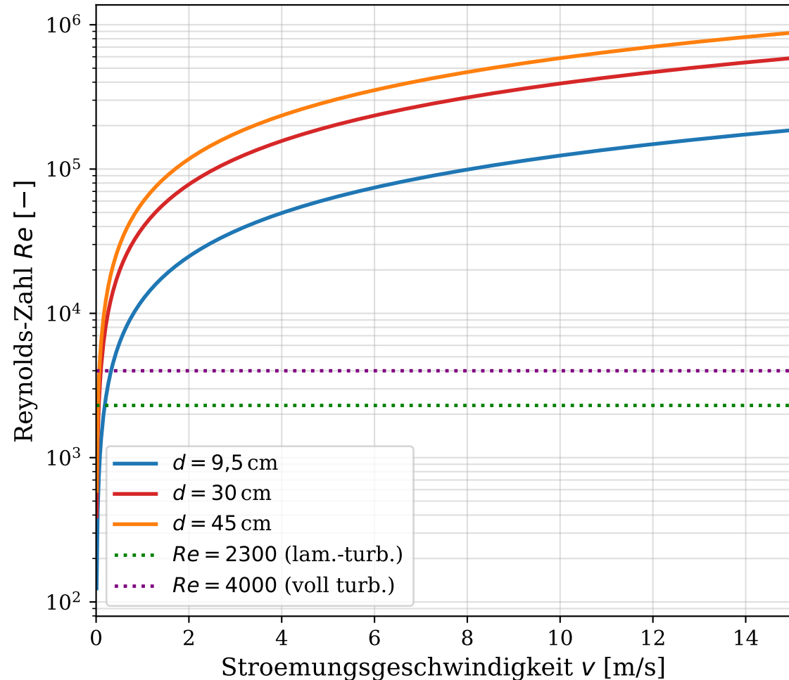
Re vs. Geschwindigkeit
