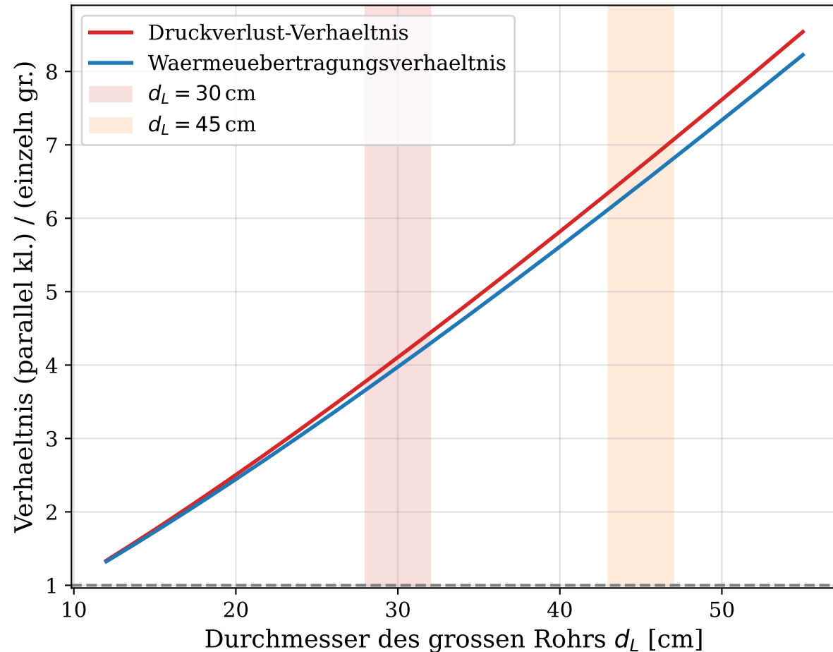
Leistungsfaeigkeitsverhaeltnis (kl. Rohre: d_s = 9.5\text{ cm} , gleiche Gesamtflaeche)
