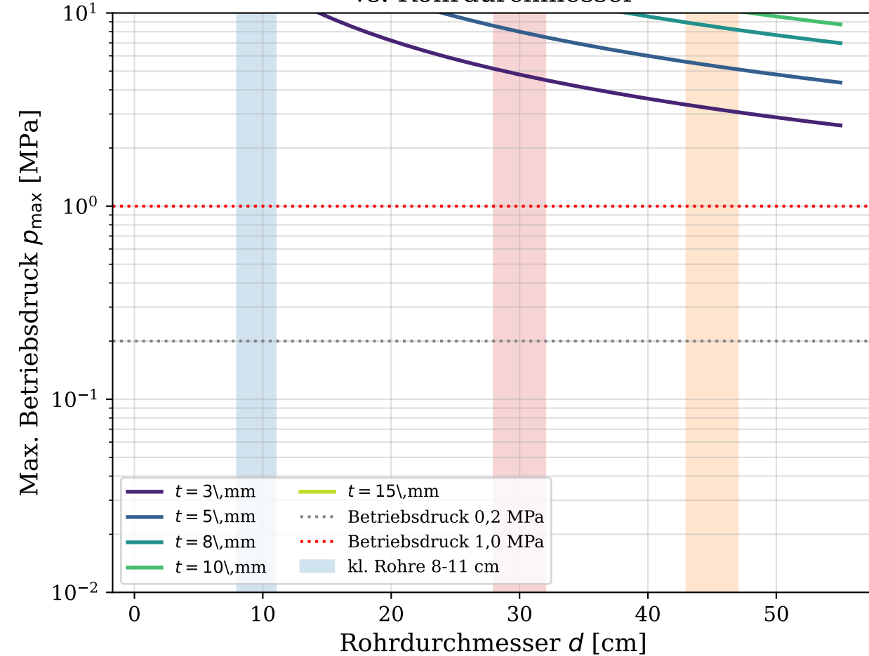
Barlow-Kurven: Zulaessiger Betriebsdruck vs. Rohrdurchmesser
