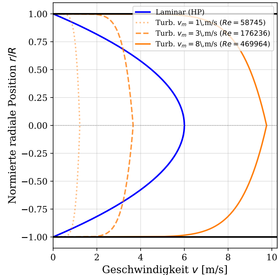
Geschwindigkeitsprofil d = 45\text{ cm}
