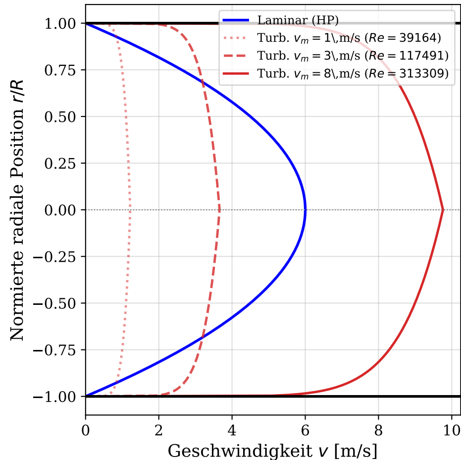
Geschwindigkeitsprofil d = 30\text{ cm}
