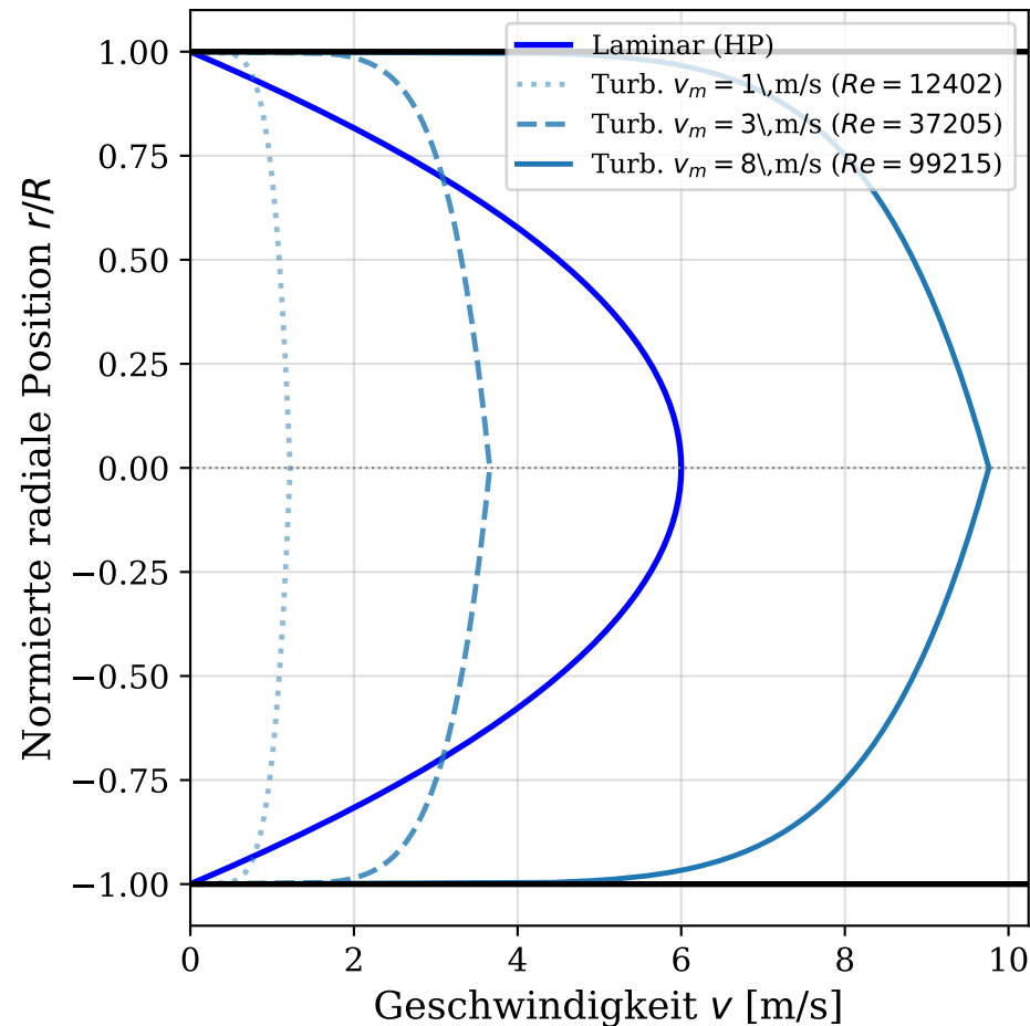
Geschwindigkeitsprofil d = 9,5\text{ cm}
