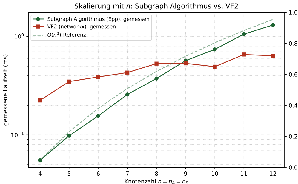
Figure 7: Gemessene Laufzeit beider Verfahren bei gemeinsam wachsendem n = n_A = n_B (5 Wiederholungen je n ), zusammen mit einer auf den ersten Messpunkt skalierten O(n^3) -Referenzkurve für den Subgraph Algorithmus.
