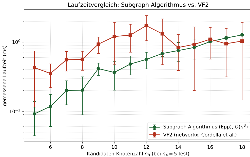
Figure 5: Gemessene Laufzeit (Mittelwert über 8 Wiederholungen, Fehlerbalken = Standardabweichung) des Subgraph Algorithmus und von VF2 in Abhängigkeit von n_B , bei festem n_A = 5 , logarithmische y -Achse.
