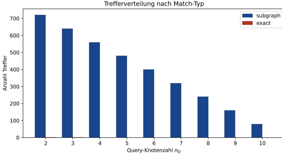
Figure 4: Verteilung der Treffertypen (exact vs. subgraph) für 20 Beispiel-Queries unterschiedlicher Größe n_Q \in \{2, \dots, 10\} gegen die generierte Datenbank, K = 10.000 .
