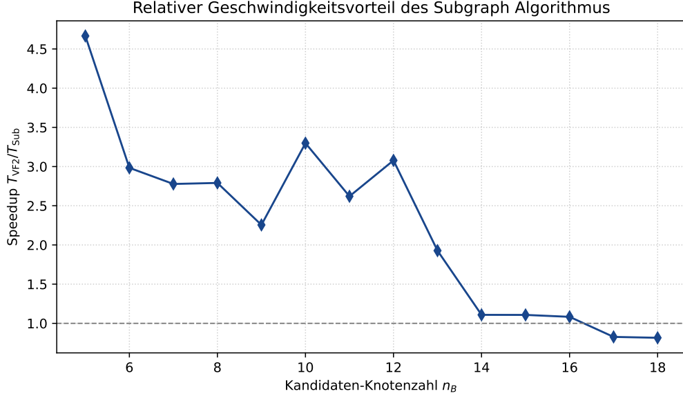
Figure 6: Speedup-Faktor T_{VF2}/T_{Sub} als Funktion von n_B (gestrichelte Linie bei 1,0: Gleichstand).
