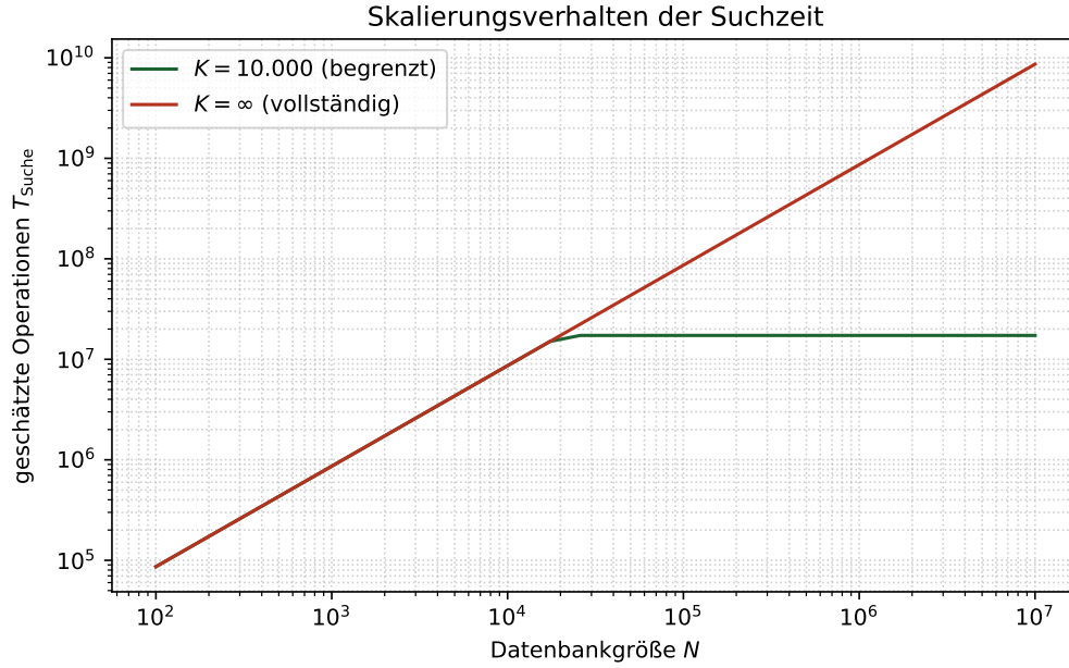
Figure 3: Geschätzte Suchzeit T_{\text{Suche}} als Funktion der Datenbankgröße N , für festes Kandidatenlimit K = 10.000 und K = \infty (volle Pipeline), gemäß Satz 2.
