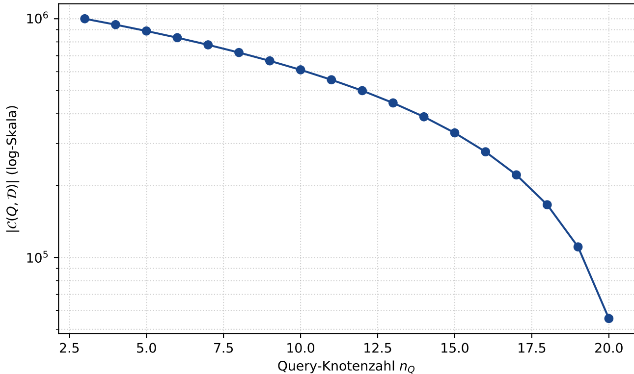
Pre-Filter-Effektivität nach Knotenzahl
