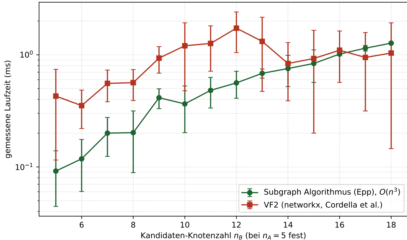
Laufzeitvergleich: Subgraph Algorithmus vs. VF2
