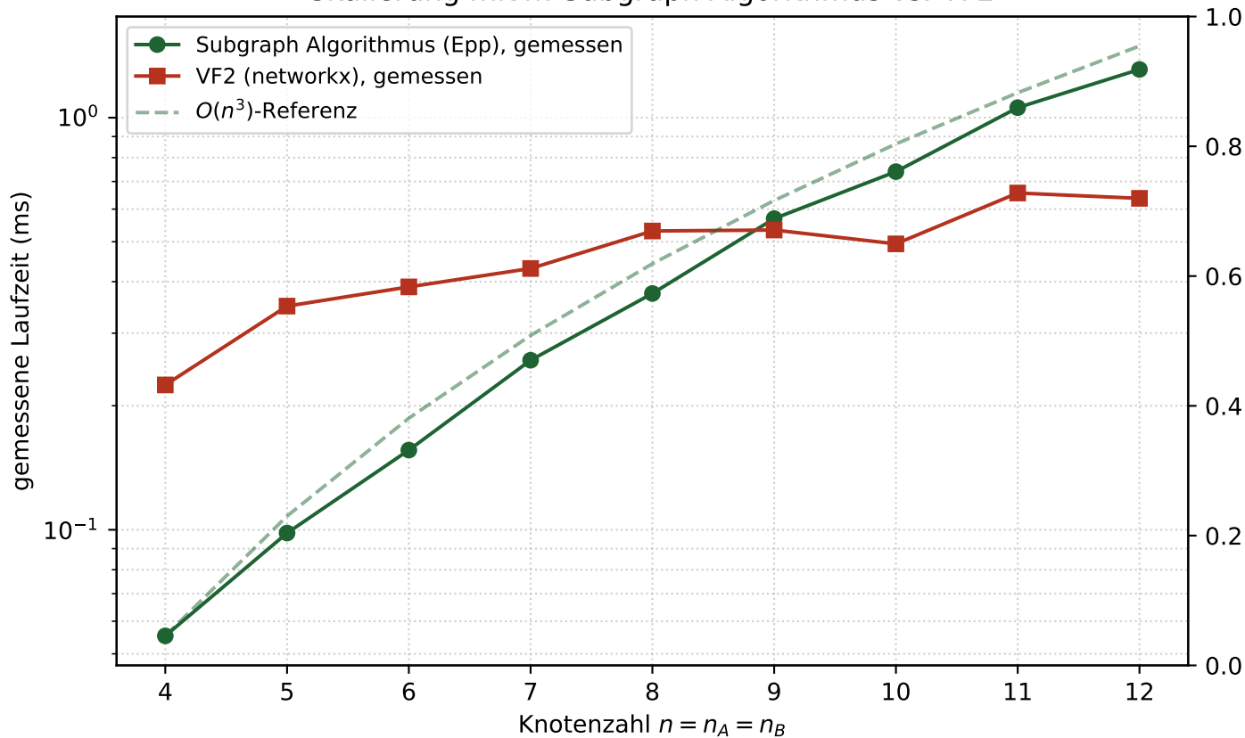
Skalierung mit n : Subgraph Algorithmus vs. VF2
