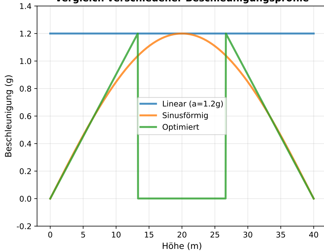
Vergleich verschiedener Beschleunigungsprofile
