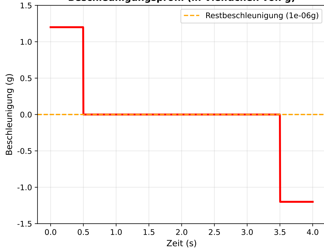
Beschleunigungsprofil (in Vielfachen von g)
