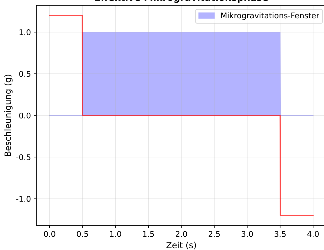
Effektive Mikrogravitationsphase
