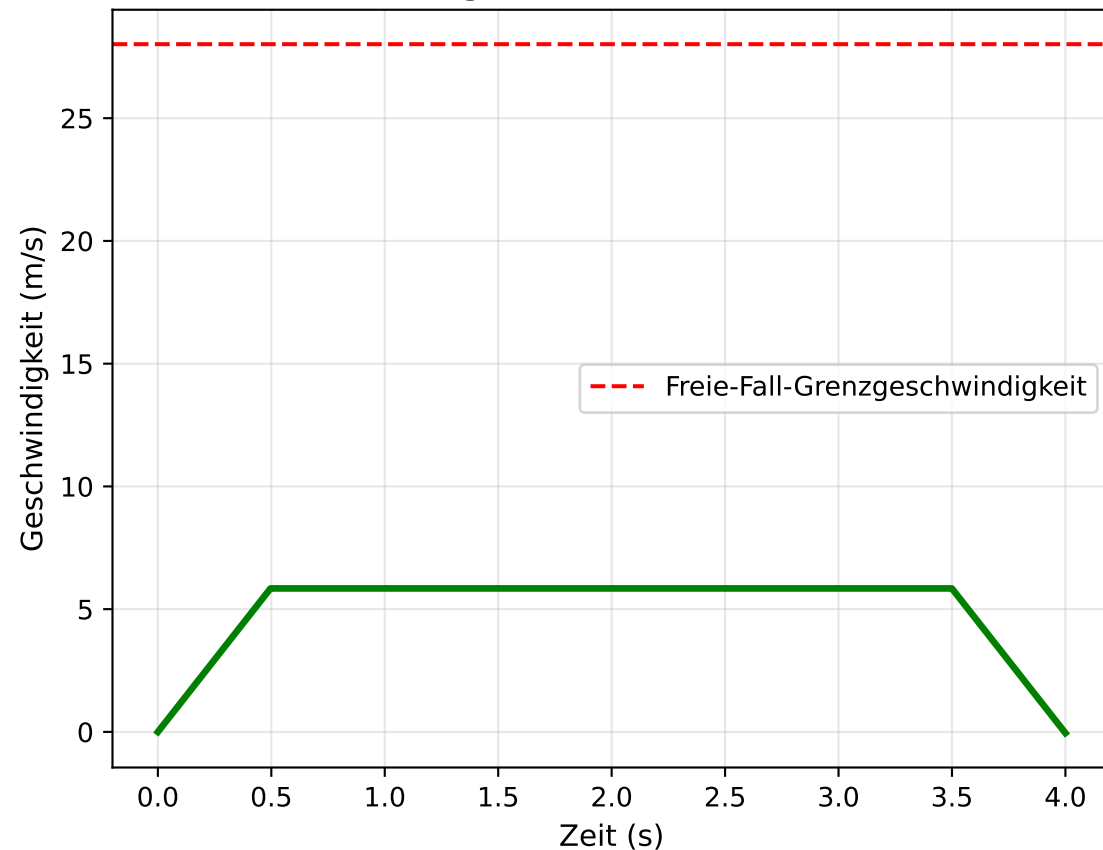
Effektive Mikrogravitationsphase
