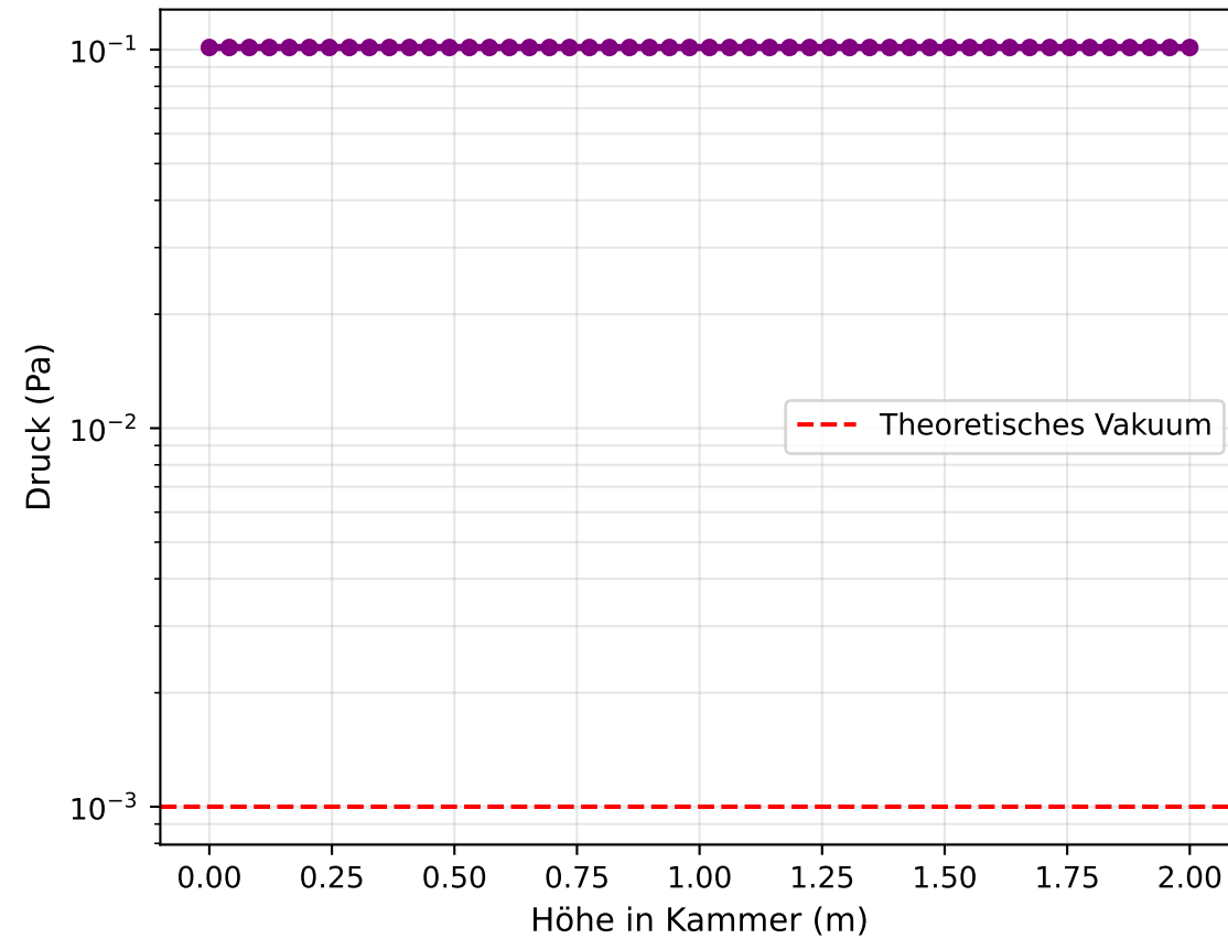
Druckverteilung in der Versuchskammer
