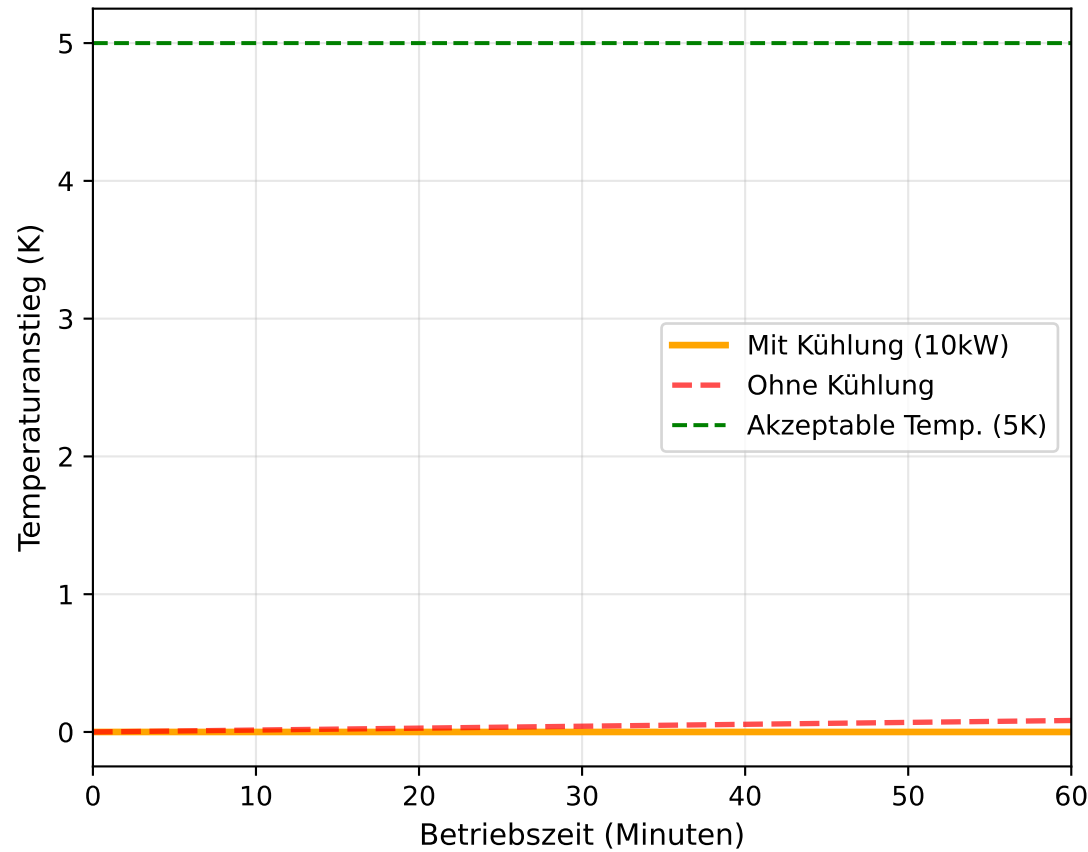
Thermische Belastung und Kühlung
