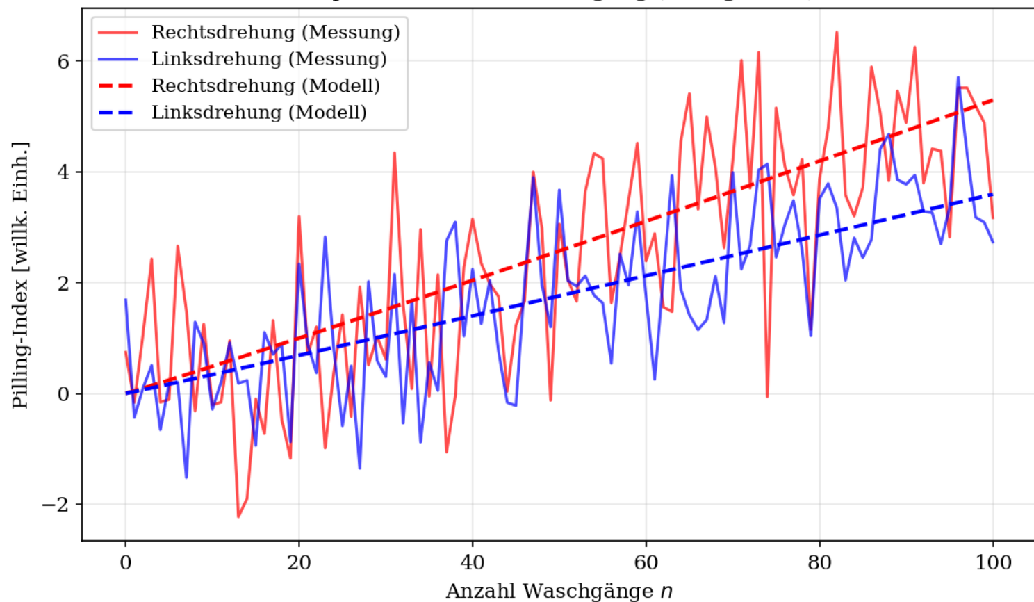
Exp. 4 – Textilfaserschädigung (Pilling-Index)
