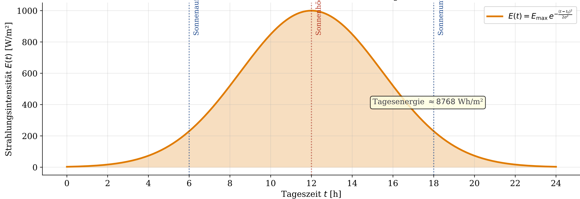
Abbildung 3: Tagesperiodische Sonnen-Energiefunktion Gauß-Modell der solaren Einstrahlung
