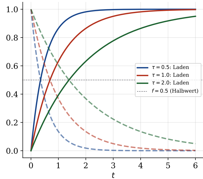
(c) RC-Lade-/Entladekurven
