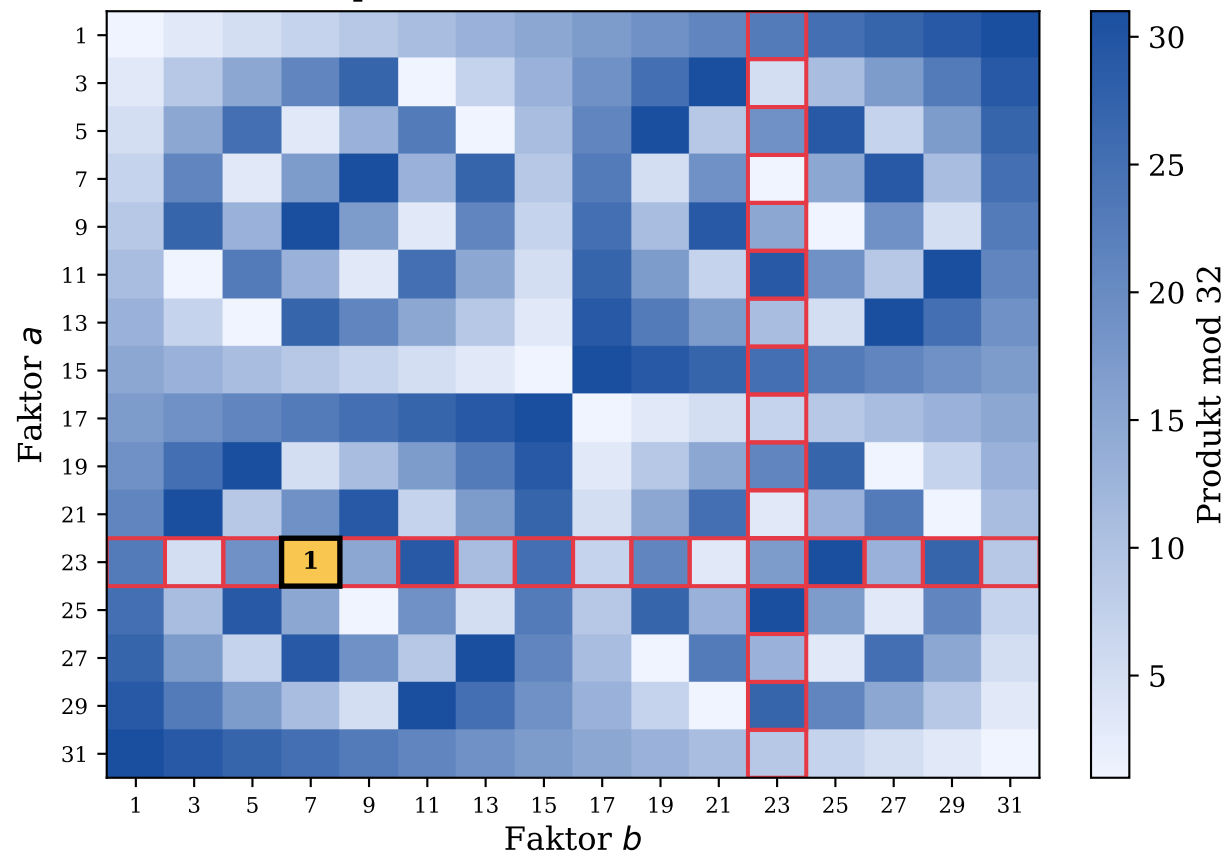
Multiplikationstabelle von (\mathbb{Z}/32\mathbb{Z})^*
