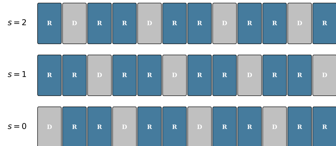
Schlüssel-Offset s \in \{0, 1, 2\} verschiebt das Dummy-Muster
