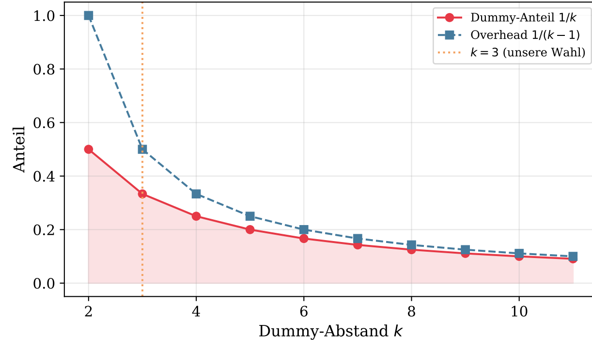
Dummy-Anteil und Traffic-Overhead in Abhängigkeit von k
