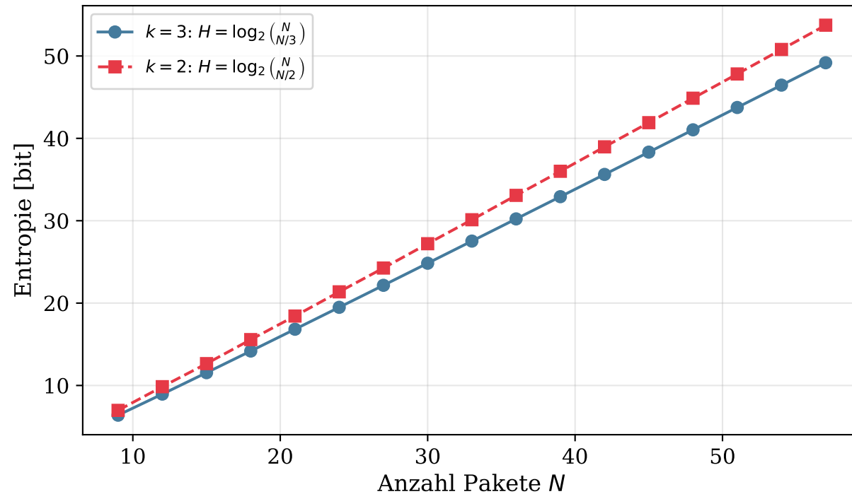
Angreifer-Entropie: Unsicherheit bei Dummy-Identifikation
