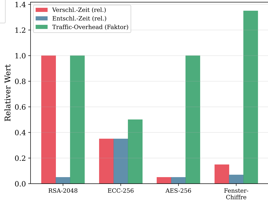
Laufzeit- und Overhead-Vergleich (normiert auf RSA-2048 = 1)
